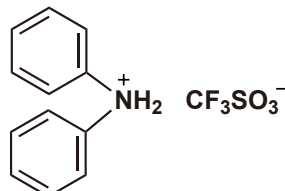
DPAT
